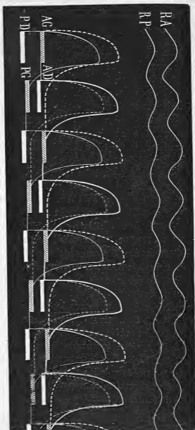
Fig. 45. — Graphiques et notation du trot d'un cheval. RA, réaction de l'avant-main. RP, réaction de l'arrière-main. AG et AD, courbes et notations des membres antérieurs. PD et PG, courbes et notations des membres postérieurs.
